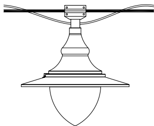
Ejemplo de montaje de WA-0 con luminaria OW, difusor cónico
