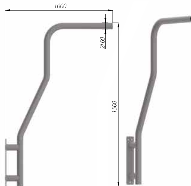
KA-19 code: 478190/C... para luminarias de parque y viales que se puedan montar en tubo Ø60
