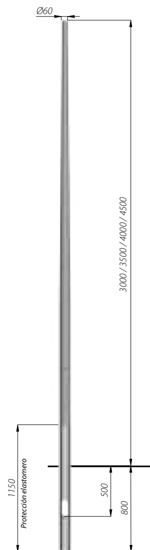
Columnas de empotrar
