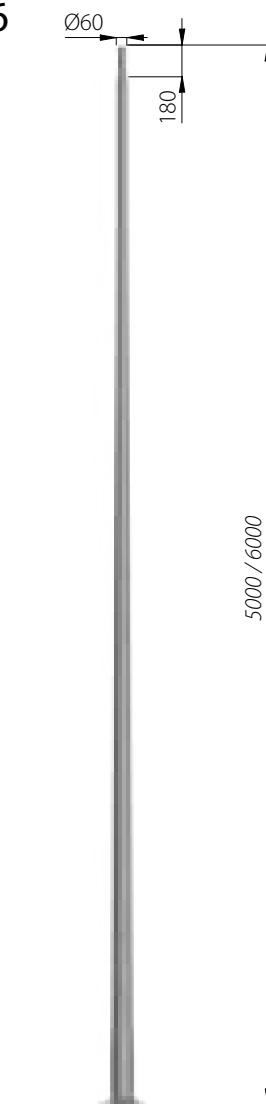
Columnas con base
