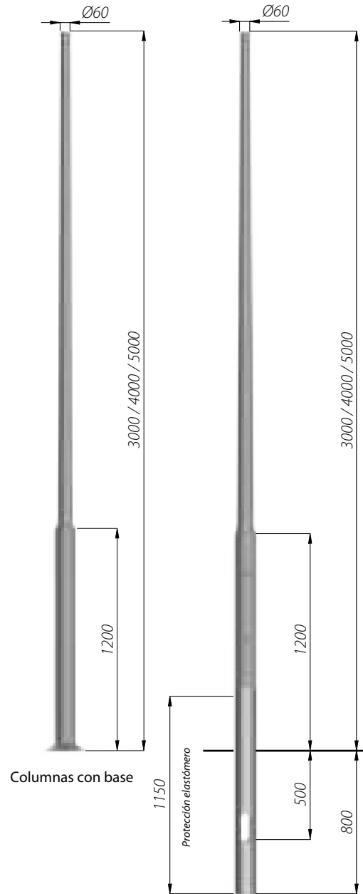
Columnas de empotrar
