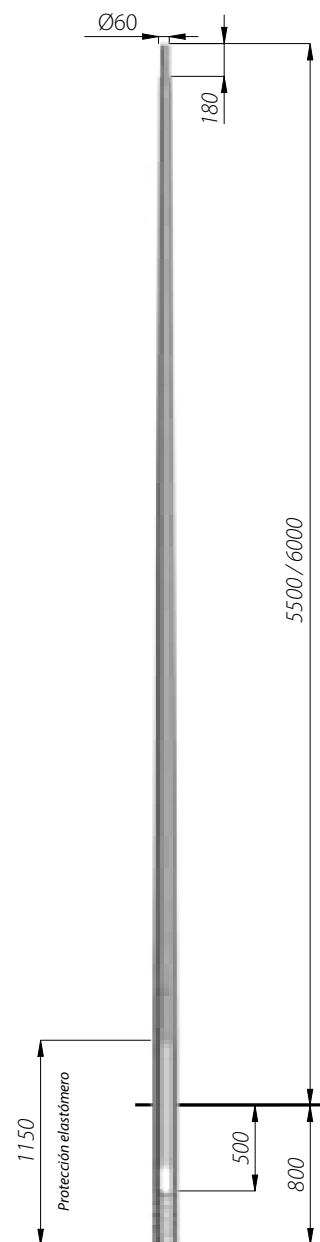
Columnas de empotrar
