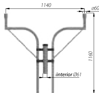
WA-5/2 code: 471052/C... luminarias: OPA-1, OP
