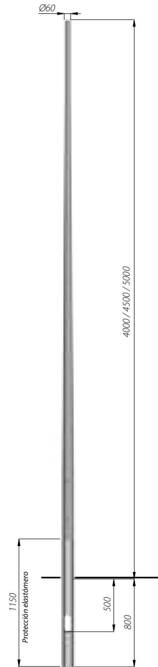
Columnas de empotrar
